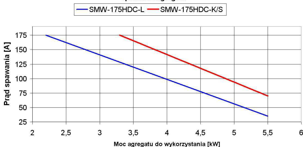
Rozdział mocy spawarki HDC - możliwość jednoczesnego wykorzystania spawarki i agregatu
